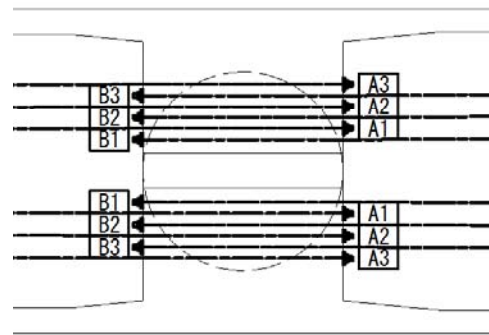
図-5 ケーブル配置平面図（柱頭部）
