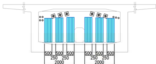
図-6 定着部補強図
