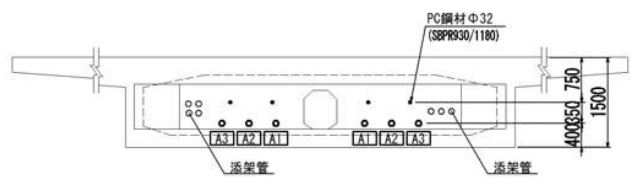
図-4 ケーブル配置断面図（ヒンジ部）
