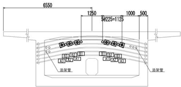
図-3 ケーブル配置断面図（定着部）
