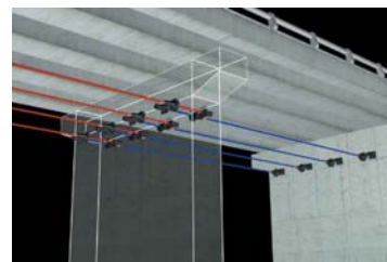
PC&PA工法イメージ
